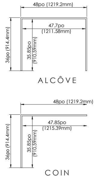
VUE DU DESSUS (ASSEMBLÉ)
